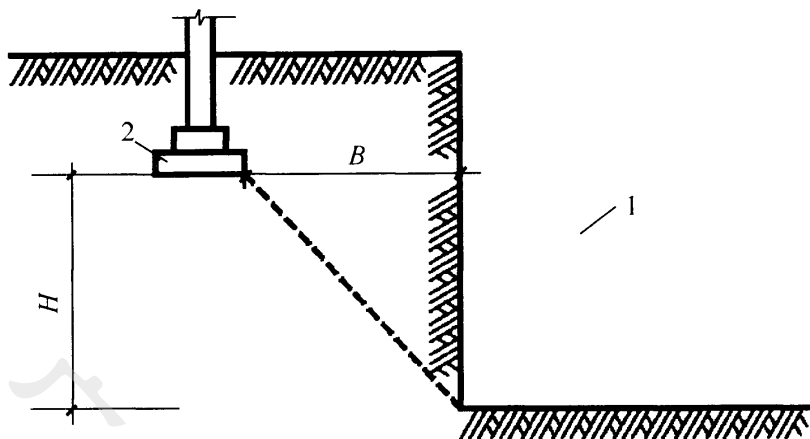
图 H.0.1-2 基坑或沟渠工程对邻近建筑基础影响的Ⅱ类影响区, B/H \leq 1 1—基坑或沟渠; 2—建筑基础
