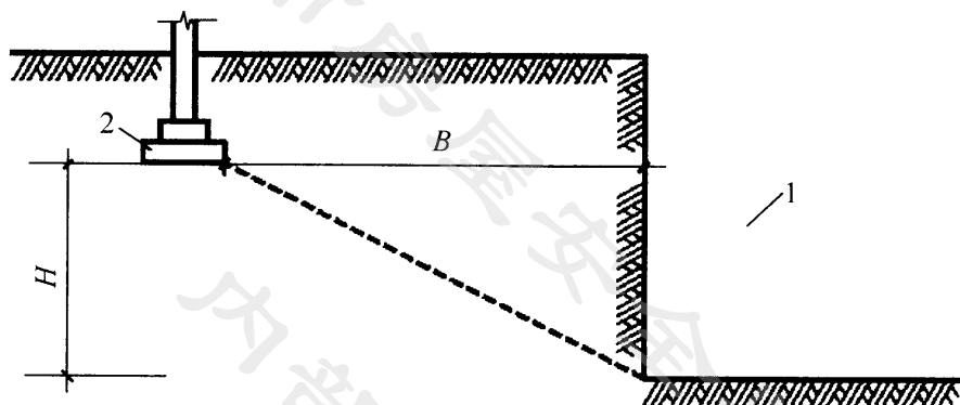
图 H.0.1-1 基坑或沟渠工程对邻近建筑基础影响的Ⅰ类影响区， B/H > 1
