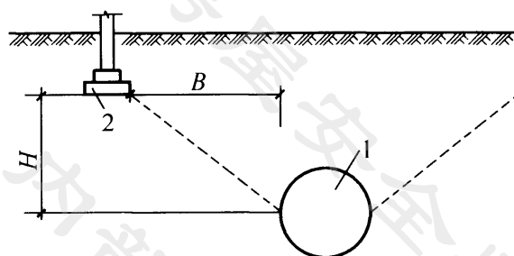
图 H.0.2-1 地下隧道工程对邻近建筑影响的Ⅰ类影响区, B/H > 1 1—地下隧道; 2—建筑基础
