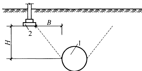
图 H.0.2-2 地下隧道工程对邻近建筑影响的Ⅱ类影响区, B/H \leq 1 1—地下隧道; 2—建筑基础
